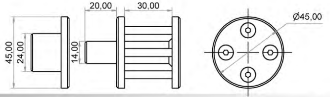
SUSTA Malzeme : Paslanmaz çelik Ağırlık : ~0,260 kg Ürün Kodu : 801.560.01
