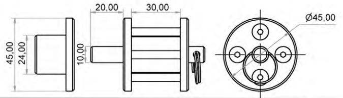
ZİNCİR ASKI Malzeme : Paslanmaz çelik Ağırlık : ~ 1kg Ürün Kodu : 801.580.01
