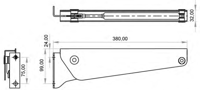
DÜZ MENTEŞE Malzeme : Paslanmaz çelik Ağırlık : ~0,255 kg Ürün kodu : 801.550.01
